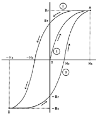
일반적인 자성체의 자성화곡선
