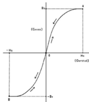
자성유체의 자성화곡선
